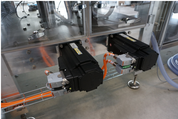
Dezentrale Servoantriebe gewährleisten einen präzisen Vorschub der Schokoladenformen. Synchronisiert werden die einzelnen Transporte durch die Motion Control IndraDrive MLC. (Bildquelle: WDS)
