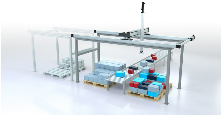
Effiziente Automatisierung in der Logistik: Mehrachssysteme, eingebunden in eine Lösung für das flexible Be- und Entladen von Paletten. (Bildquelle: Bosch Rexroth AG)
