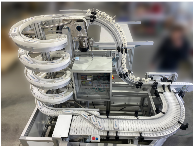
Spiralny system transportowy oparty na komponentach systemu przenośników łańcuchowych VarioFlow. (Źródło zdjęcia: Bosch Rexroth AG)
