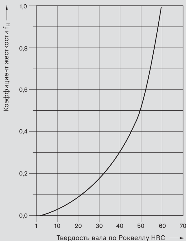
Диаграмма коэффициентов жесткости f_H
