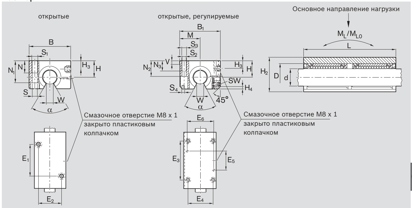
Размеры (мм)
