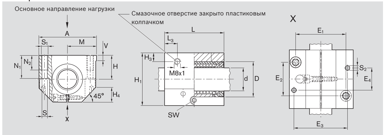
Размеры (мм)
