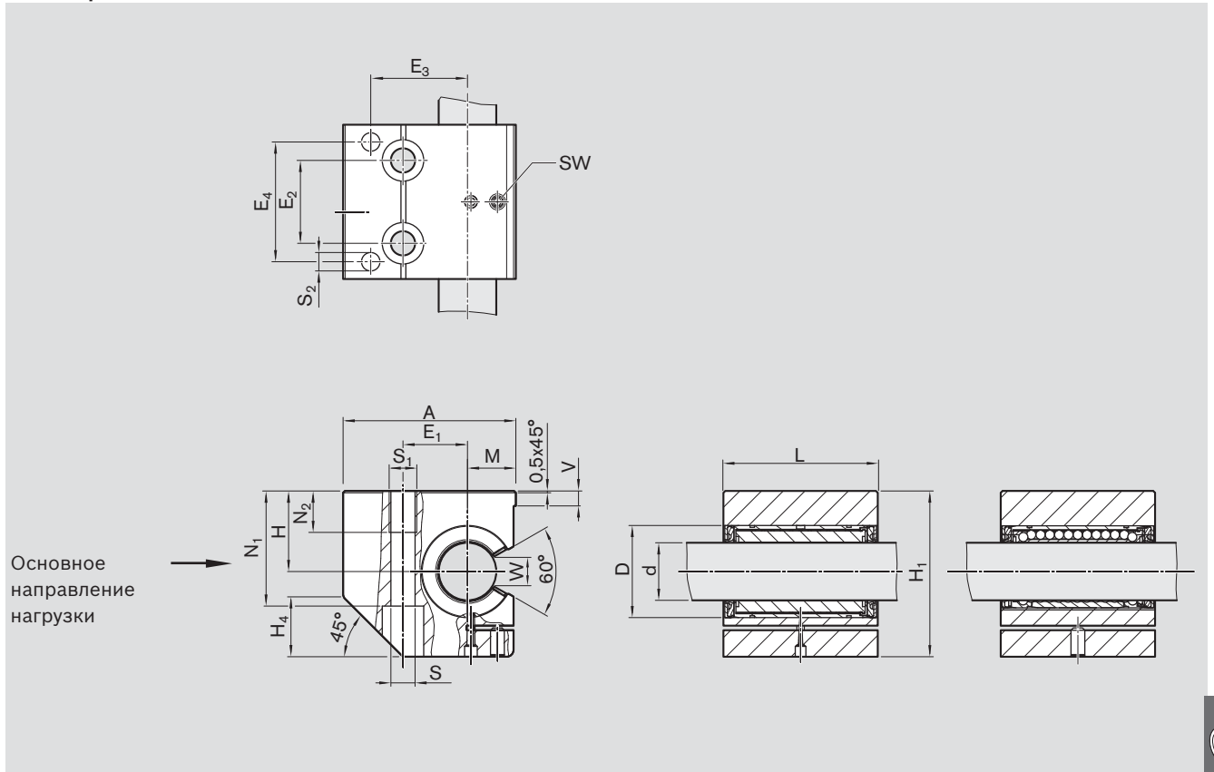
Размеры (мм)
