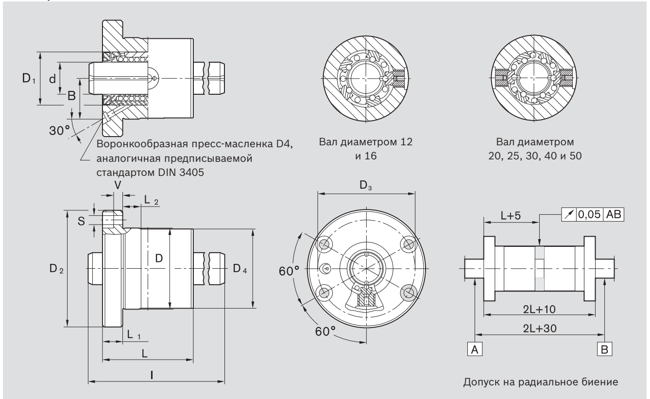
Размеры (мм)
