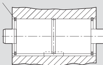
Предохранительное кольцо DIN 472
