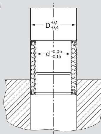
Монтажная оправка
