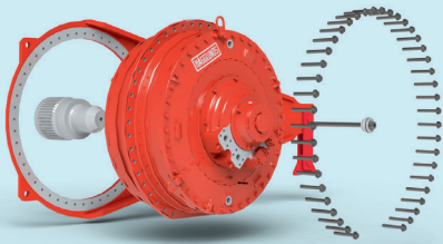
▲ Hägglands MB 1150/1600
